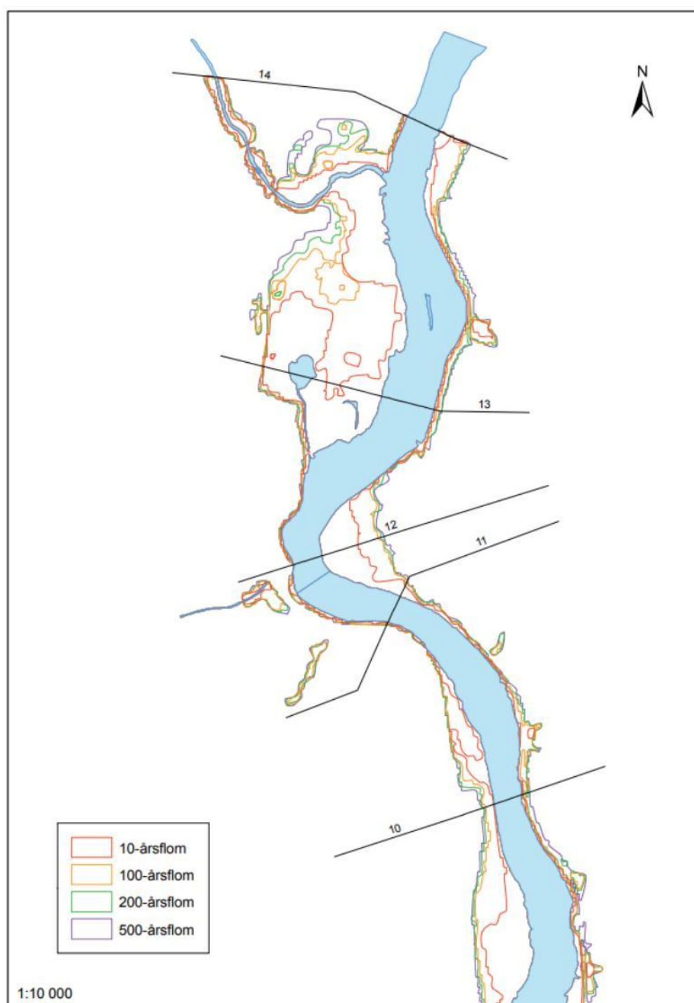
Figur 1.1: Oversiktsbilde over beregnede tverrprofiler fra NVEs rapport Flomsonekart, Delprosjekt Mosby . Mosby Ringvei 28 ligger like ved tverrprofil nr. 13.
